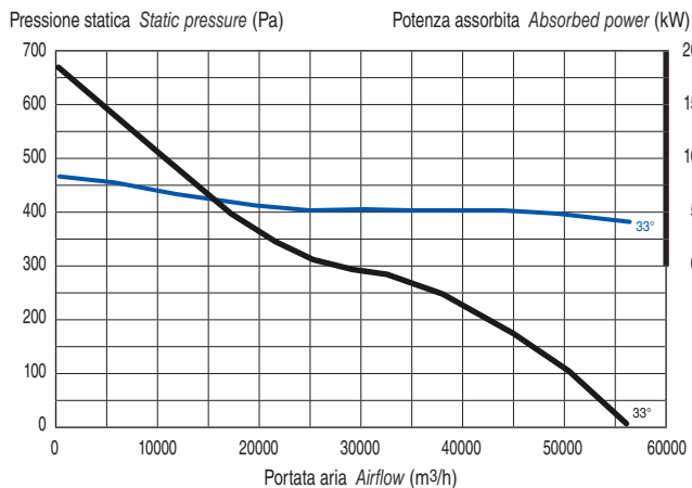
mod. 1126/C · 5,5 kW Potenza installata Motor power
