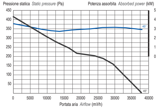
mod. 1006/A · 2,2 kW Potenza intallata Motor power
