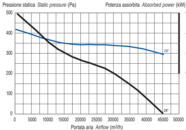
mod. 1126/B · 4 kW Potenza installata Motor power
