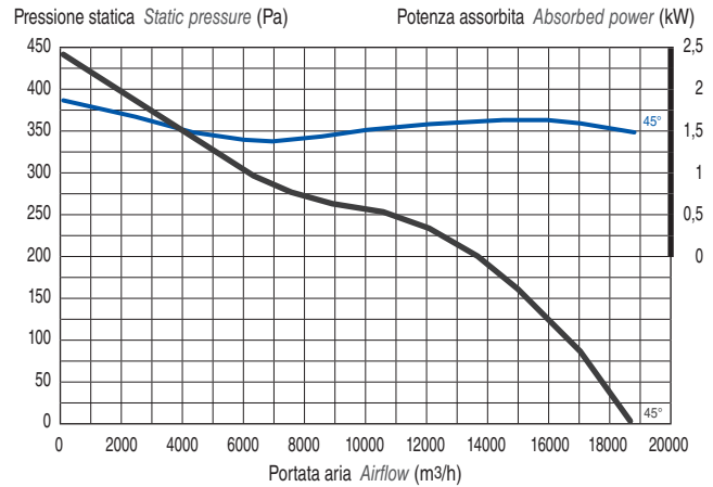
mod. 714/A · 2,2 kW Potenza installata Motor power
