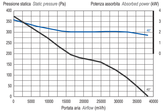
mod. 1006/B · 3 kW Potenza intallata Motor power
