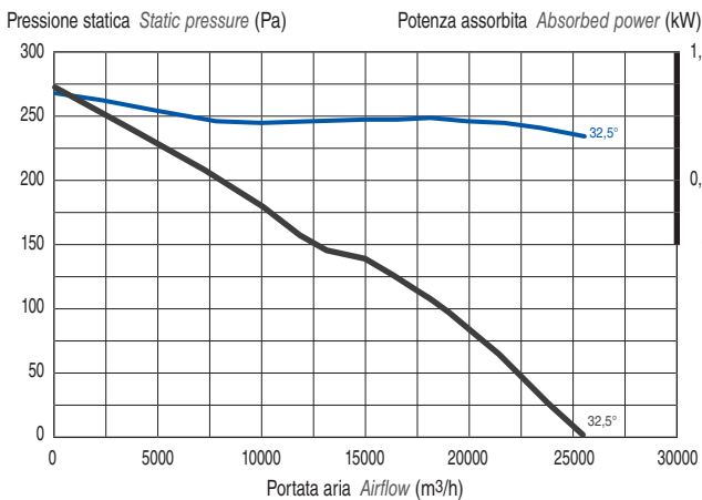
mod. 906/B · 2,2 kW Potenza intallata Motor power
