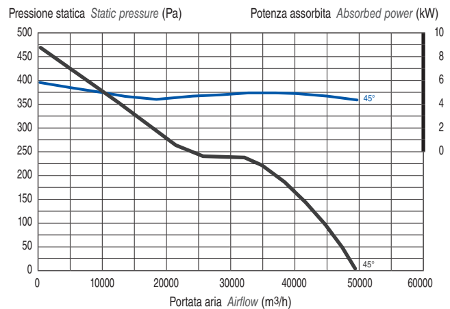
mod. 1006/C · 5,5 kW Potenza intallata Motor power
