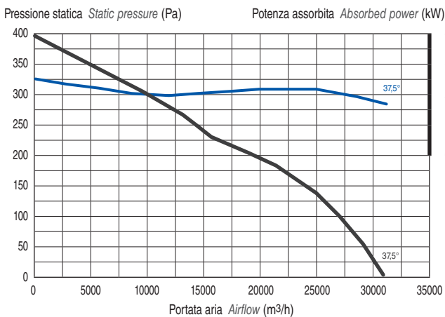
mod. 906/B · 2,2 kW Potenza intallata Motor power
