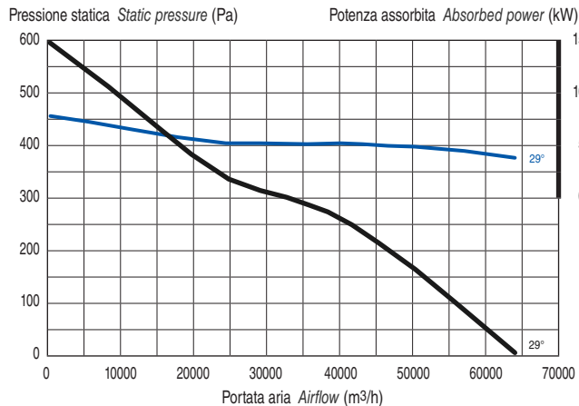
mod. 1256/B · 7,5 kW Potenza installata Motor power
