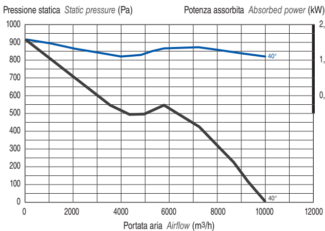
mod. 402/B · 2,2 kW Potenza installata Motor power
