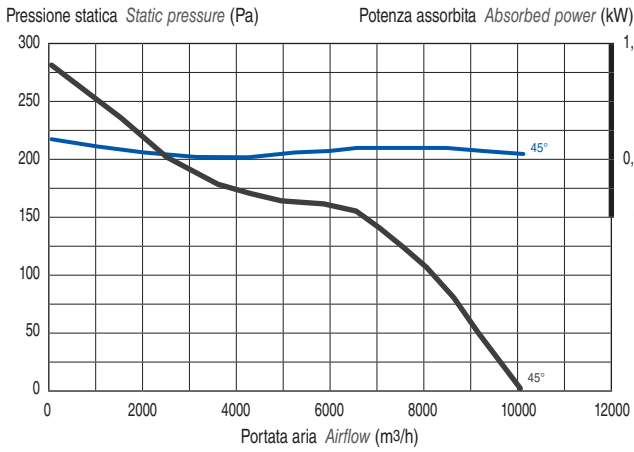
mod. 564/A · 0,75 kW Potenza installata Motor power
