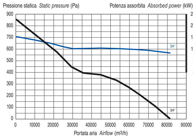
mod. 1256/C · 11 kW Potenza installata Motor power
